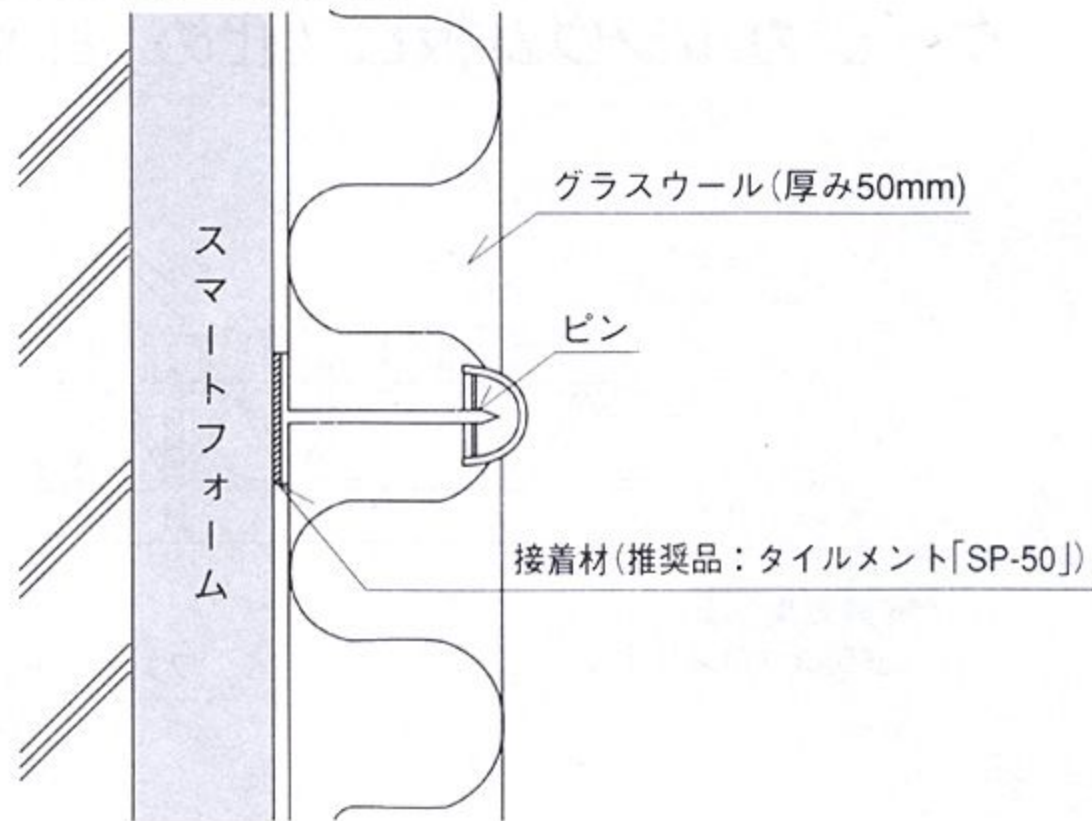
2. ピン止め仕様収まり図
