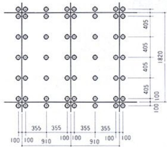
1. グラスウール用ピン間隔(例)
