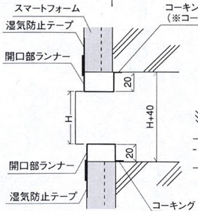
開口部ランナー取付図
