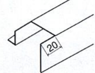
開口下部ランナー加工図
