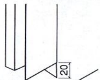
開口上部ランナー加工図
